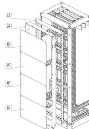
Пластронная система
