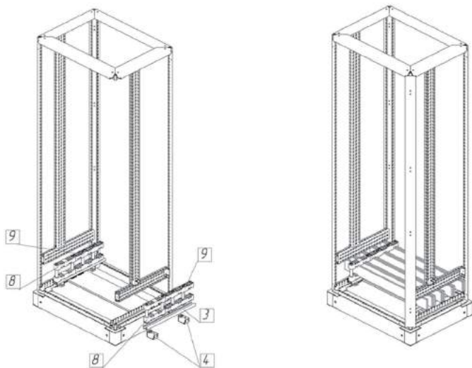
Шинодержатели
