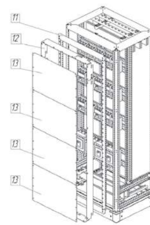
Пластронная система
