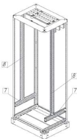
Шинные сборки
