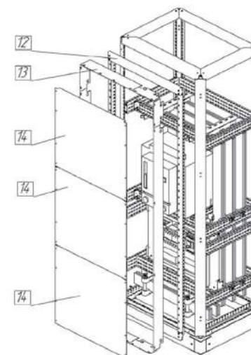
Пластронная система
