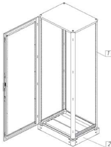
Распределительный шкаф
