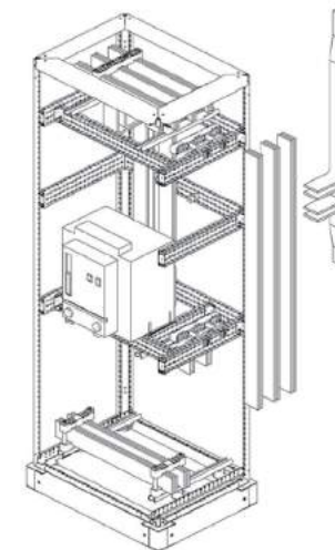
Шинные сборки
