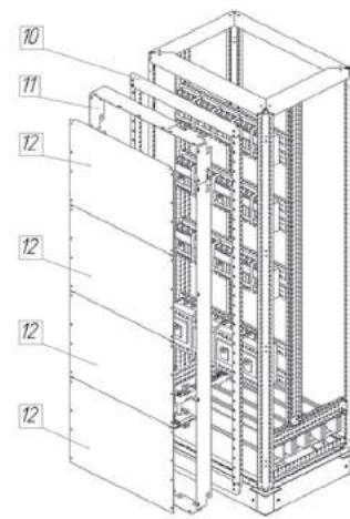
Пластронная система
