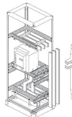
Шинные сборки
