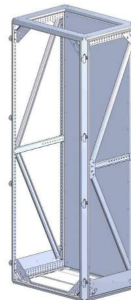
Сейсмостойкий комплект IK 01 EQ
