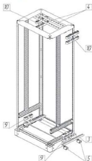
Шинодержатели
