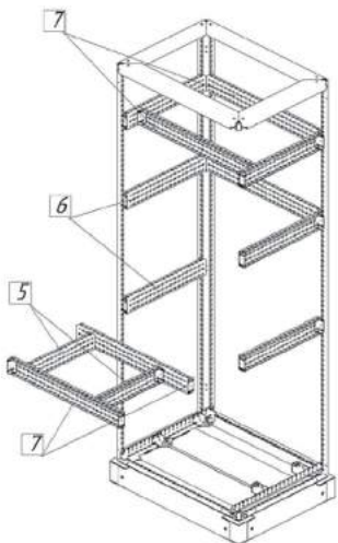
Система профилей
