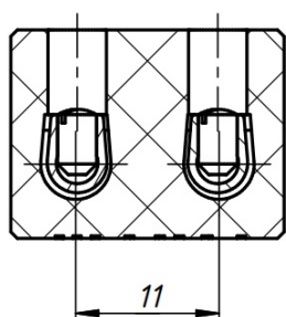
A-A (2:1)
