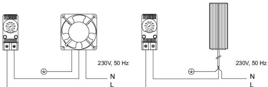
Терморегулятор TS 6.230 NOD
